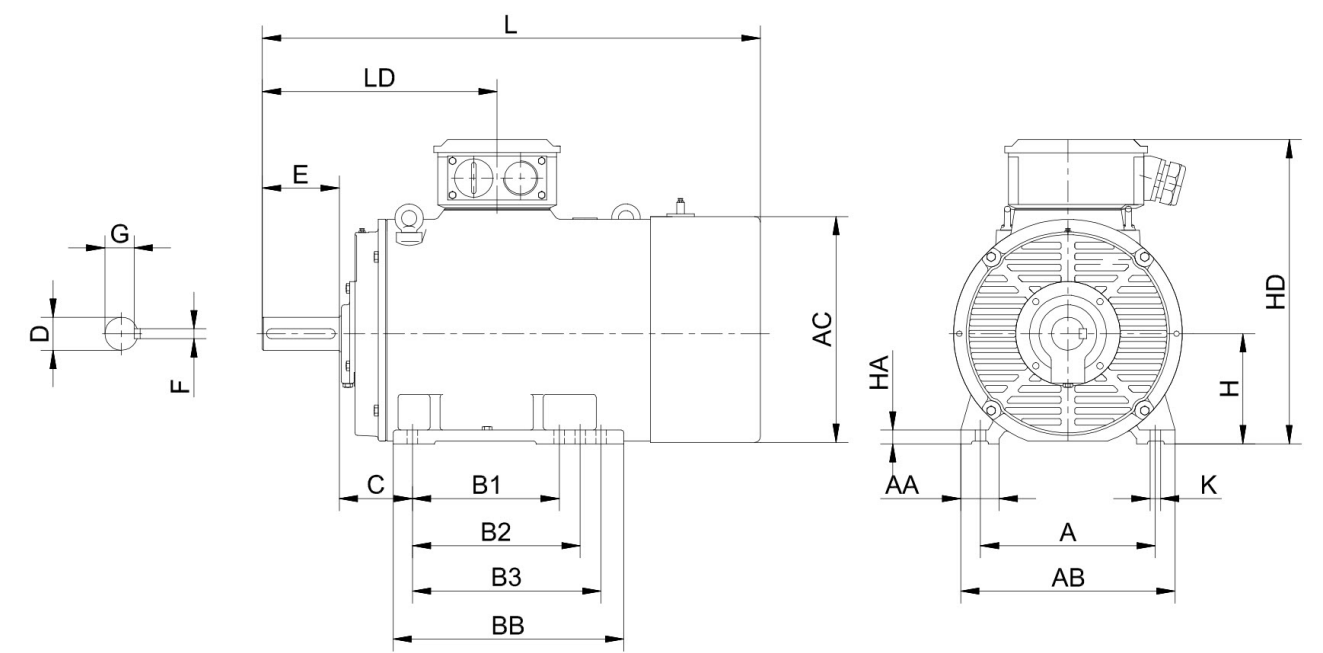
OMD IE3 DIMENSIONS FRAME 160-250
